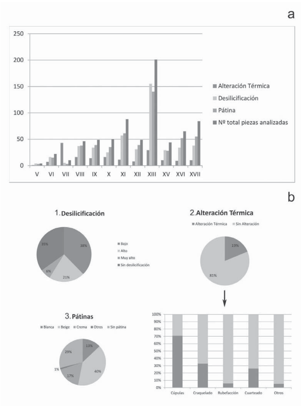
Figura 3. Gráficos con las alteraciones presentes en el conjunto lítico analizado. a) Presencia de las alteraciones y su distribución estratigráfica en relación al número total de piezas analizadas en cada Unidad Estratigráfica. b) Proporción de las alteraciones en el total del conjunto analizado. b.1 porcentaje de las piezas con desilicificación y grado de ésta. b.2 Porcentaje de alteración térmica sobre el total (arriba) y presencia de fenómenos de alteración térmica en base al total de material termoalterado (abajo). b.3. Porcentaje de material patinado y coloración de la pátina
