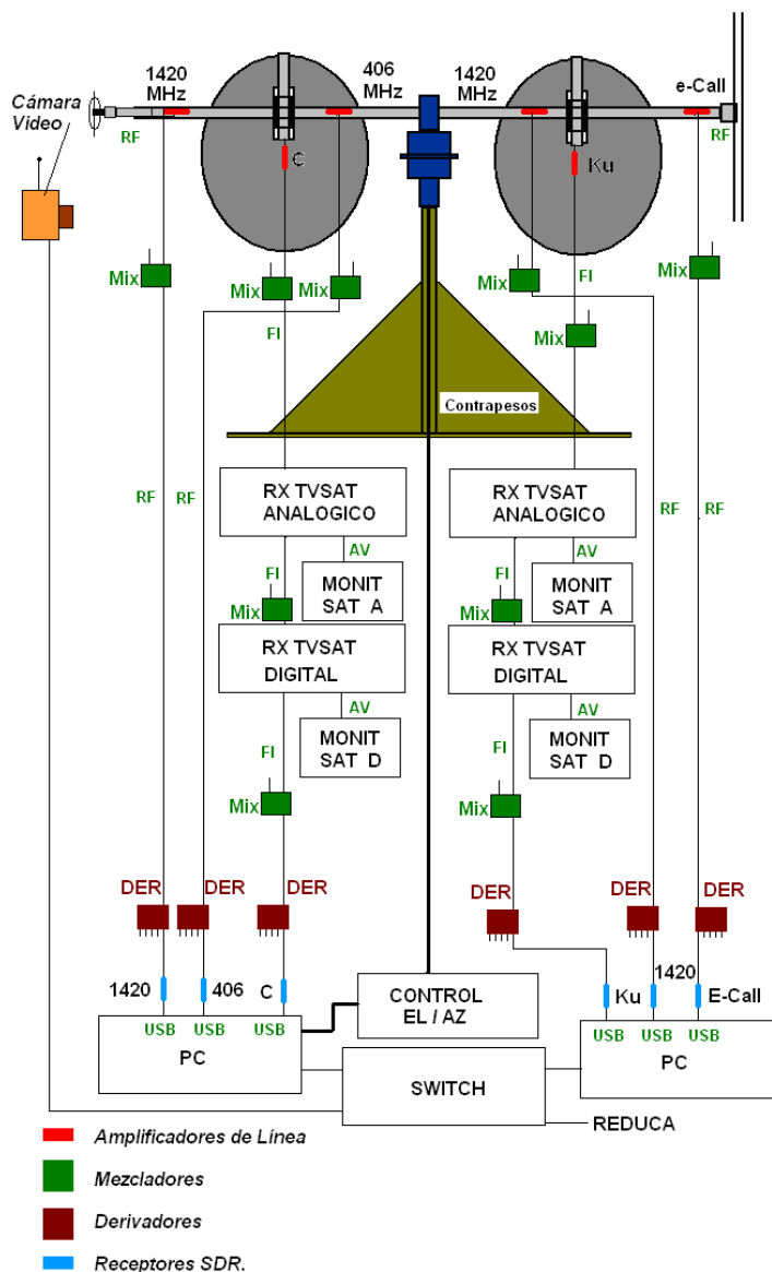
Figura 1. Demostrador de Conceptos de Radiofrecuencia EAC10 Patentado por la UCA.
